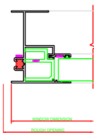
402 JAMB SERIES: 3500
